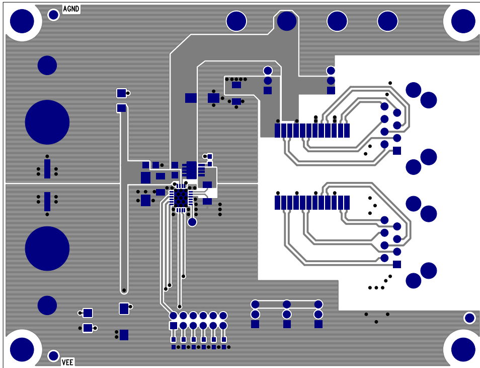
Top Layer
