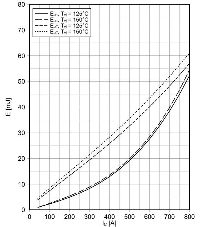
Schaltverluste IGBT, T1 / T4 (typisch) switching losses IGBT, T1 / T4 (typical)
