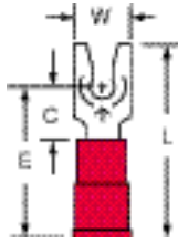
MVU18-4FL Stud Size: 4 Wire Range: 22-18
