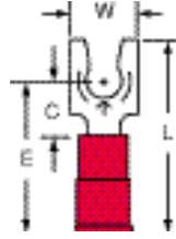
MVU18-8FL Stud Size: 8 Wire Range: 22-18
