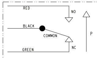
SPDT
