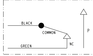
SPNC
