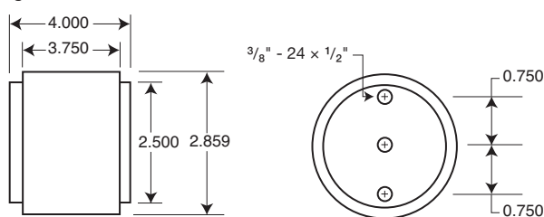
Fig. 3: 800A
