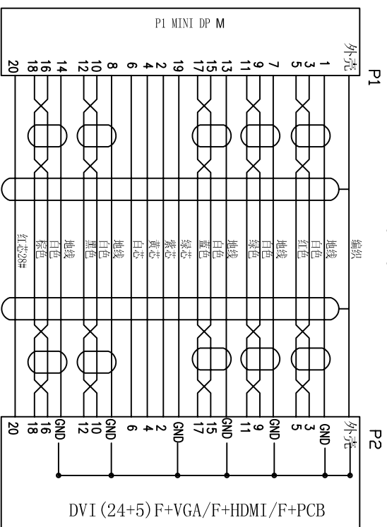
1. Wiring Diagram.
