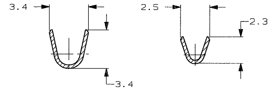
SEZIONE B-B (SECTION B-B)
