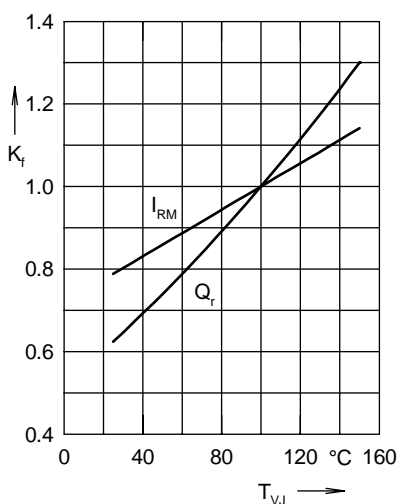
Fig. 4 Dynamic parameters K_r , I_{RM} versus T_{VJ}
