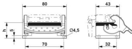
Maßzeichnung
